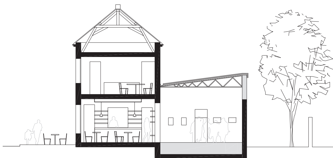
Coupe transversale
