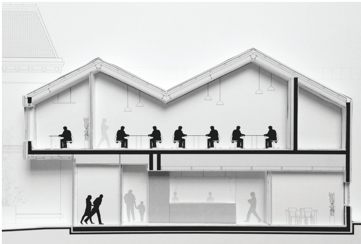
Bas-relief, coupe transversale
